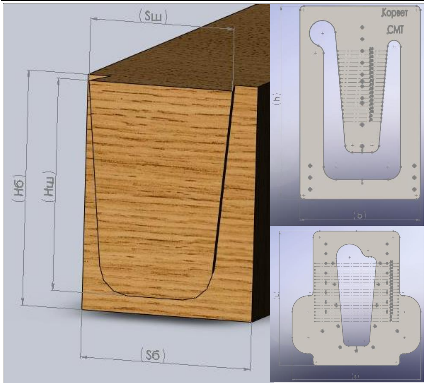
Габариты шипового соединения
